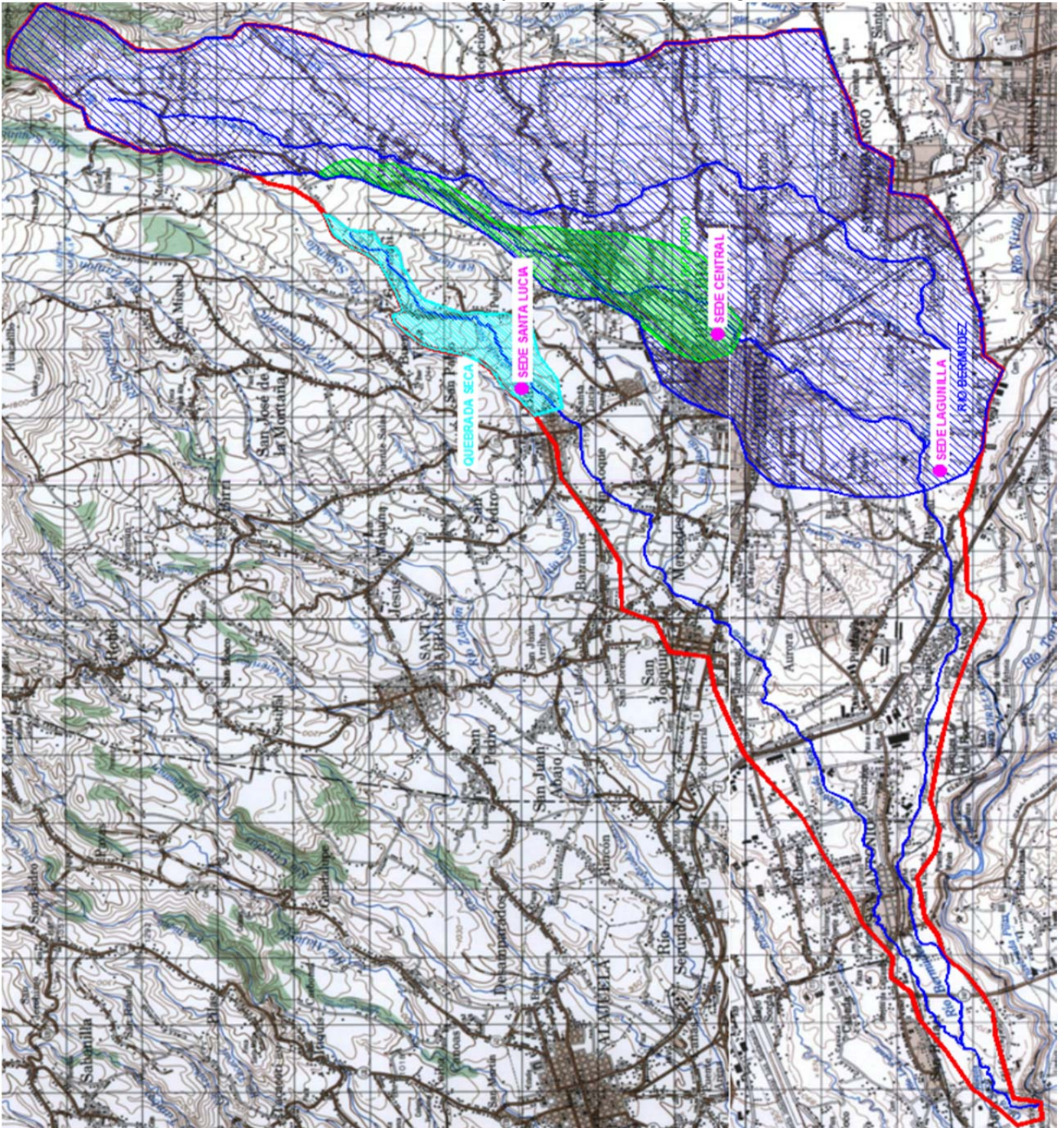
Figura N° 7.3. PGA Proyecto Construcción de Edificio de Procesos Artísticos. Ubicación de las Cuencas de Estudio y las AP según Hoja Cartográfica.
