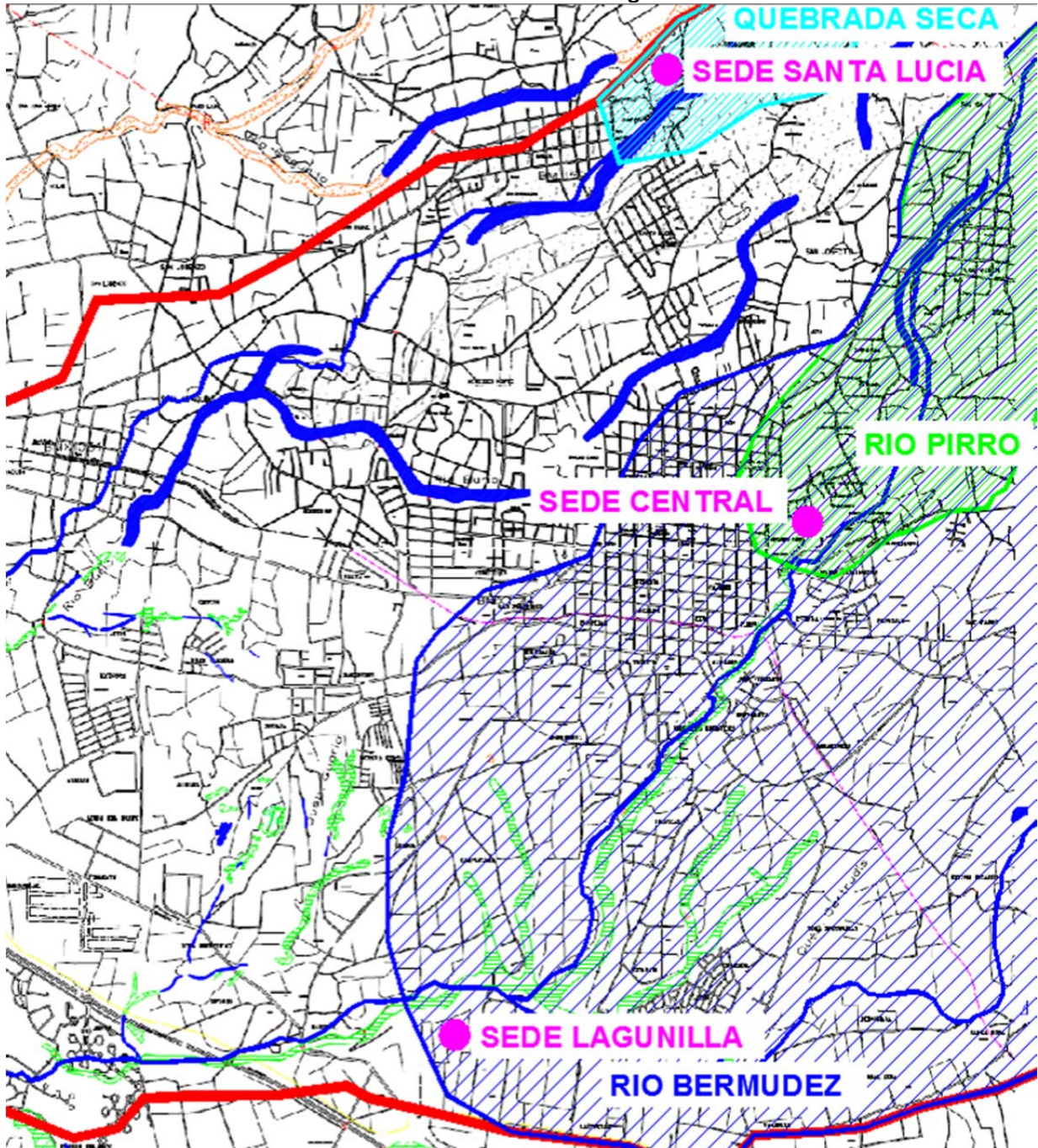
Figura N° 7.4. PGA Proyecto Construcción de Edificio de Procesos Artísticos. Ubicación de la Cuenca de Estudio y las AP sobre el Mapa de Riesgo de Inundación de la Comisión Nacional de Emergencias.
