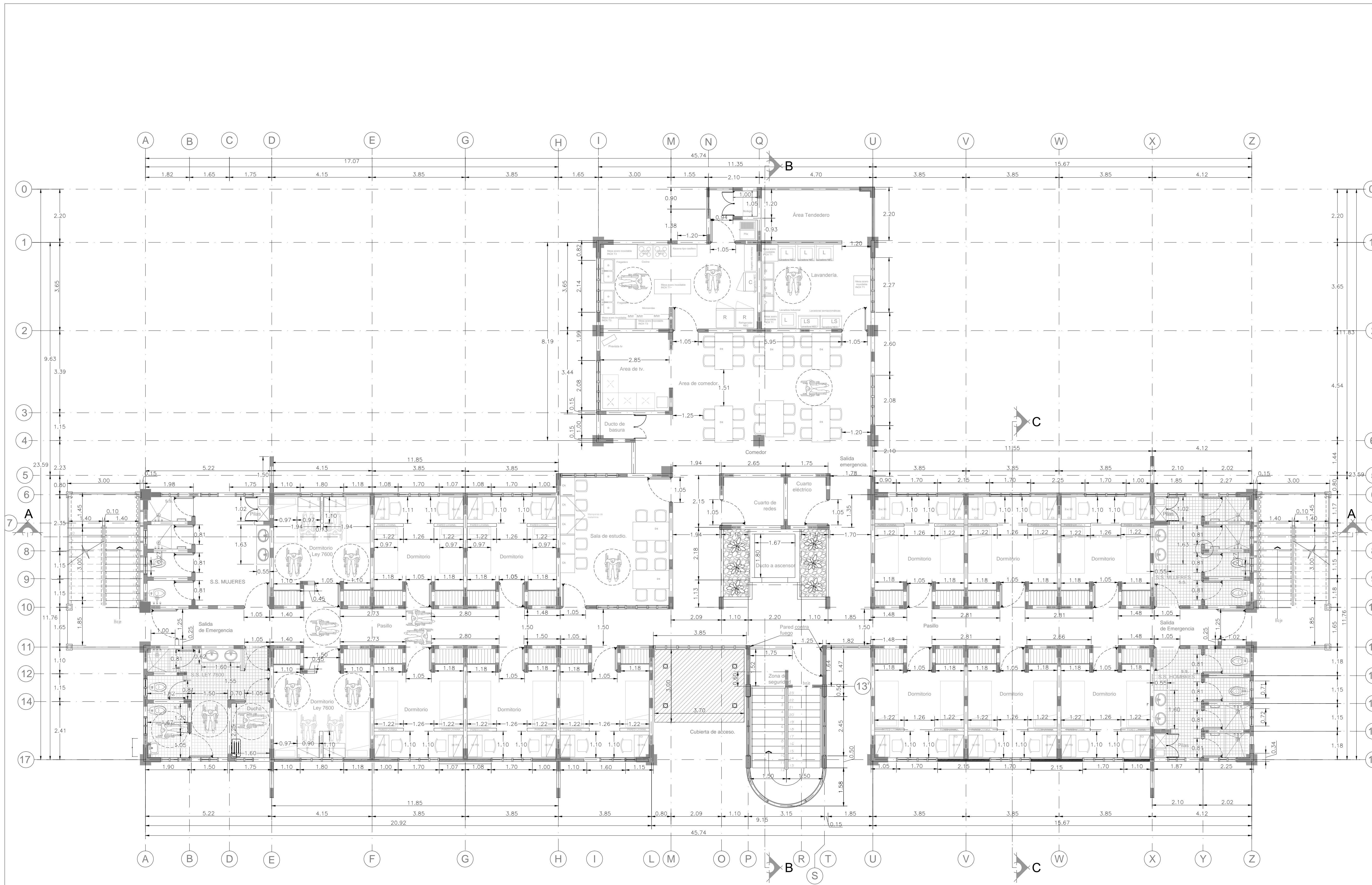
PLANTA DE DISTRIBUCION ARQUITECTONICA ACOTADA NIVEL 2. RESIDENCIAS ESTUDIANTILES LIBERIA. ESCALA 1/75
