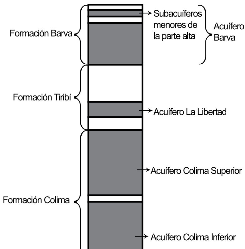
Figura 2 Columna geológica simplificada, a escala libre, de la cuenca del río Virilla.
