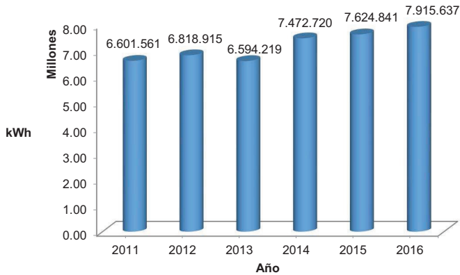
Figura 4. Demanda de energía eléctrica (kWh/año) de la UNA para los años 2011-2016.
