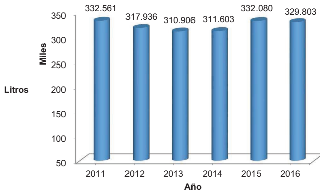
Figura 6. Gasto de combustible diésel (L/año) de la UNA para los años 2011-2016.
