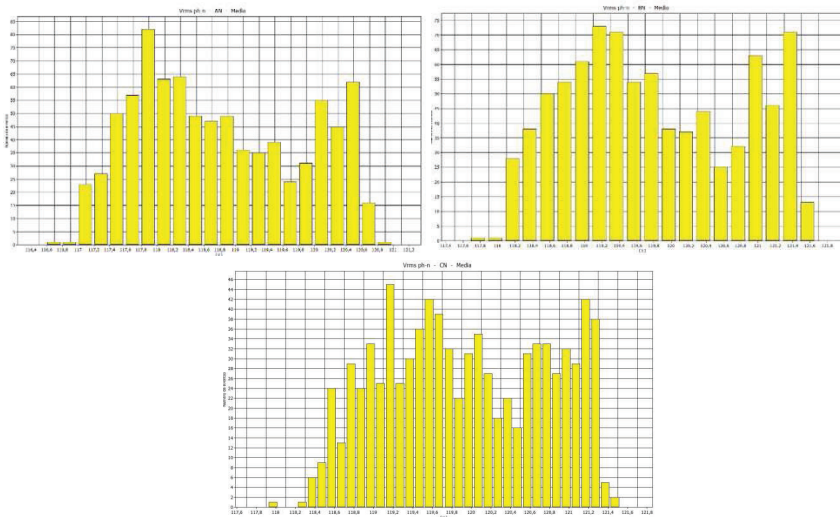
Figura 16. Consumo energético en voltaje (V) del Edificio de Usos Múltiples, Universidad Nacional.
